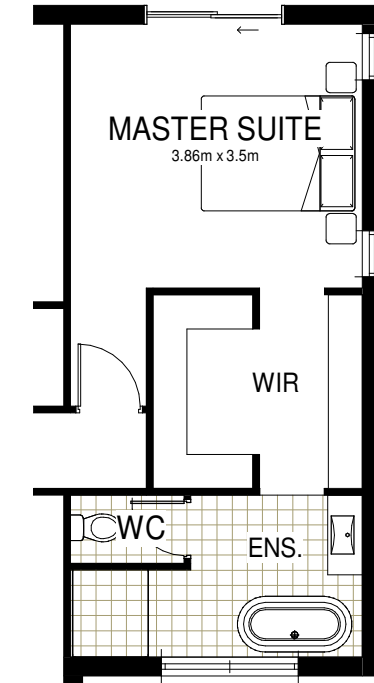
MASTER SUITE OPTIONAL LAYOUT
