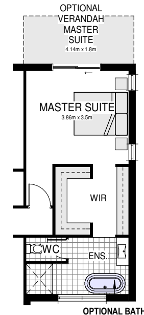
MASTER SUITE OPTIONAL LAYOUT
