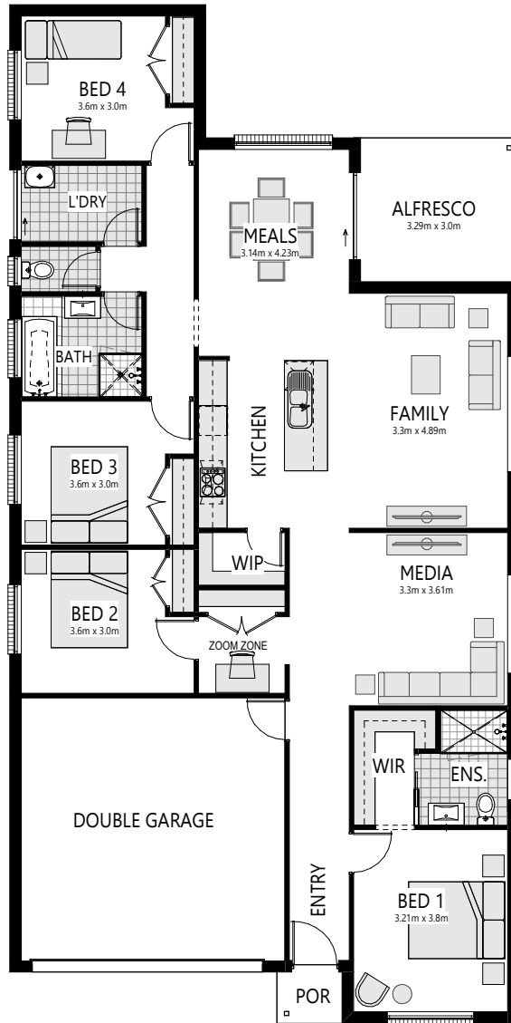
1 FLOOR LAYOUT SCALE: 1 : 100
